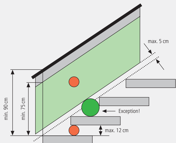
Rampe d'escalier
